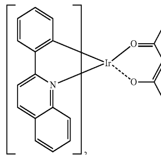
Ir(pq) 2 (acac)
