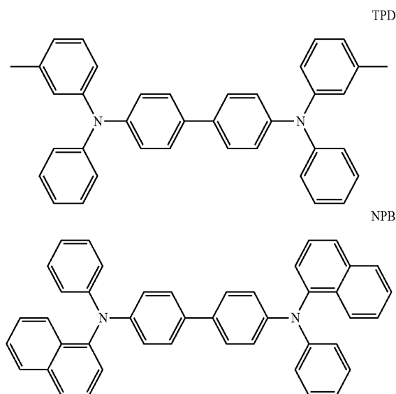
TPD
