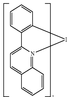
Ir(2-phq) 3
