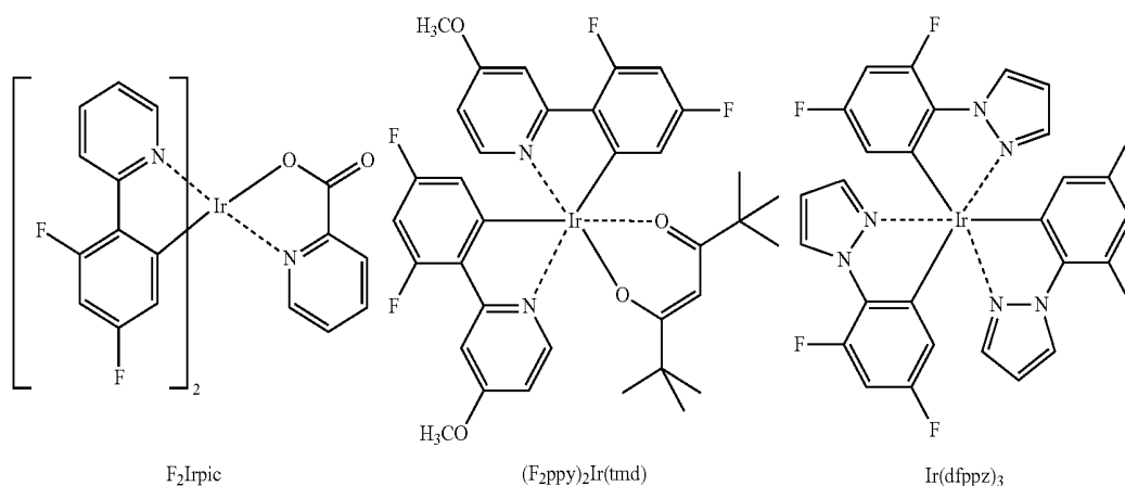
Ir 2 Ipic
